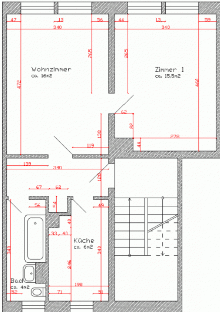
2-Raumwohnung ca. 47m2
